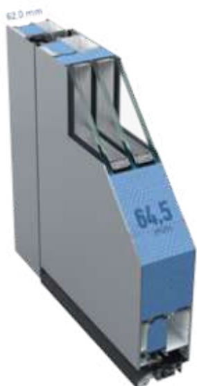
ERT|75 Flacher Rahmen Aussen
