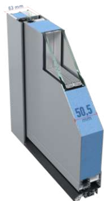
ERT|50 Flacher Rahmen Aussen
